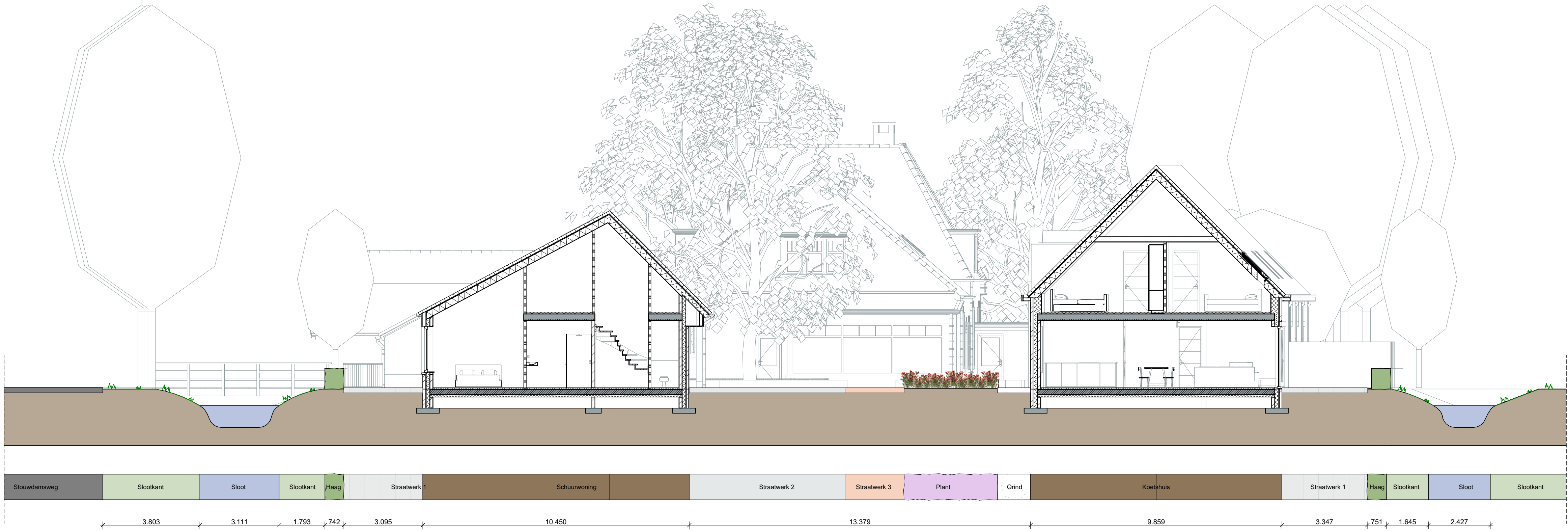
DOORSNEDE 1-1
