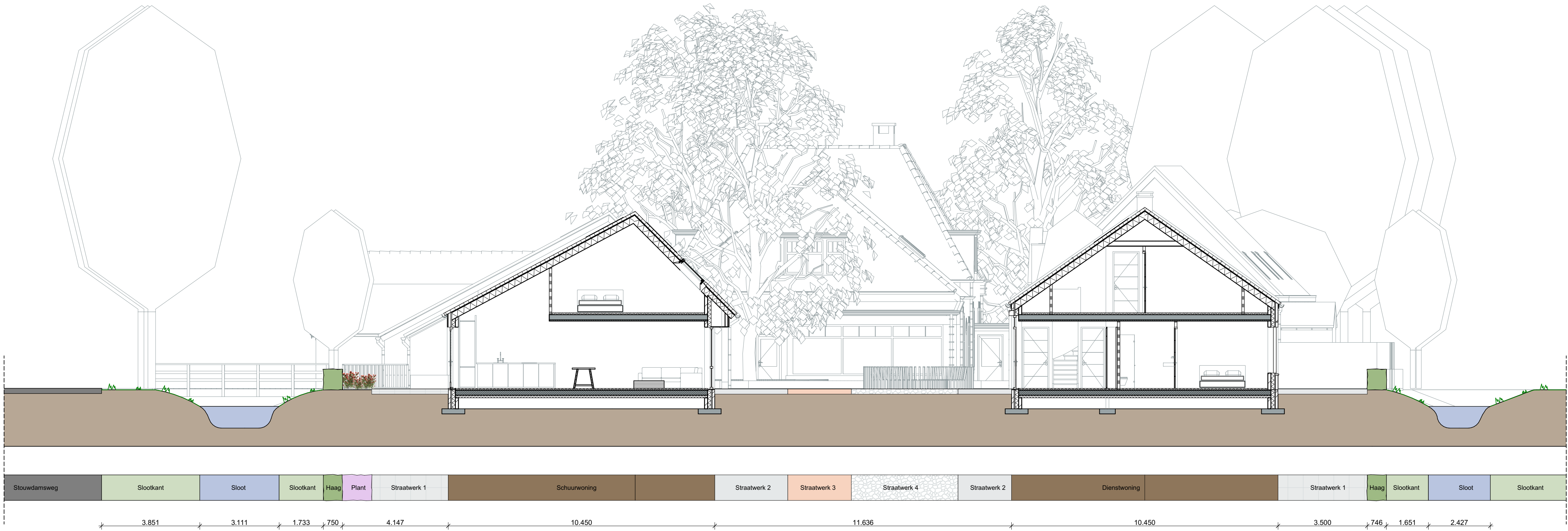
DOORSNEDE 2-2
